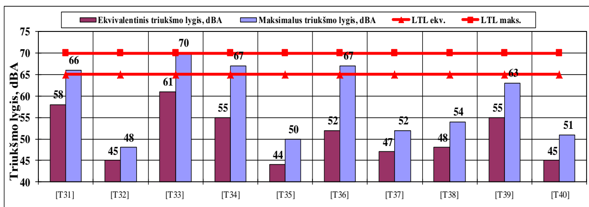
4.18 pav. Ekvivalentiniai ir maksimalūs triukšmo lygiai dienos metu T31–T40 tyrimo vietose
