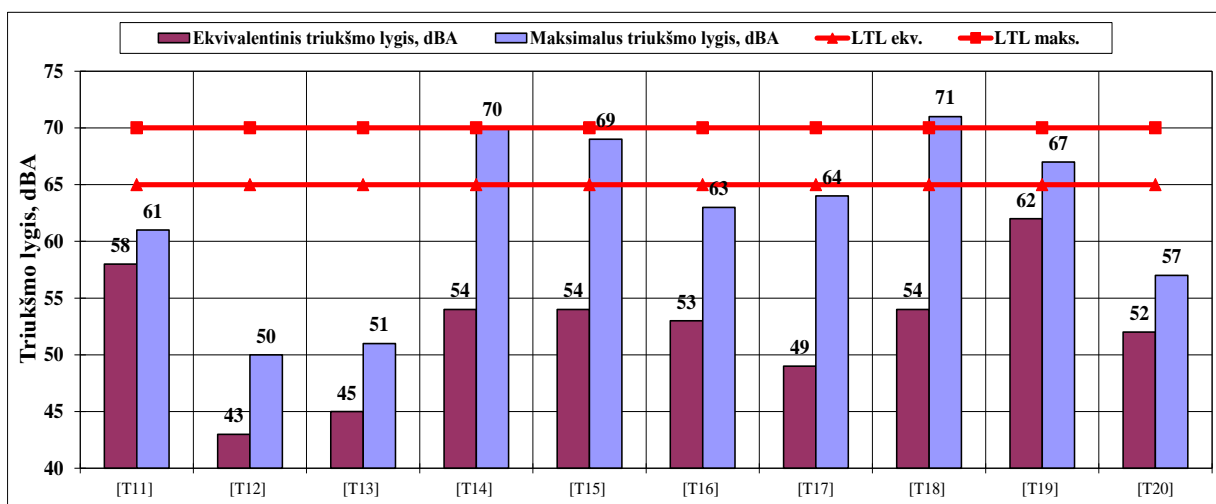
4.4 pav. Ekvivalentiniai ir maksimalūs triukšmo lygiai dienos metu T11–T20 tyrimo vietose
