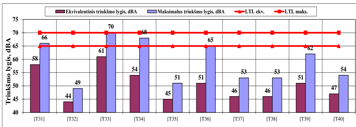
4.6 pav. Ekvivalentiniai ir maksimalūs triukšmo lygiai dienos metu T31–T40 tyrimo vietose
