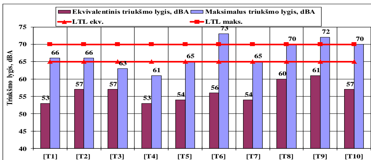
4.15 pav. Ekvivalentiniai ir maksimalūs triukšmo lygiai dienos metu T1–T10 tyrimo vietose
