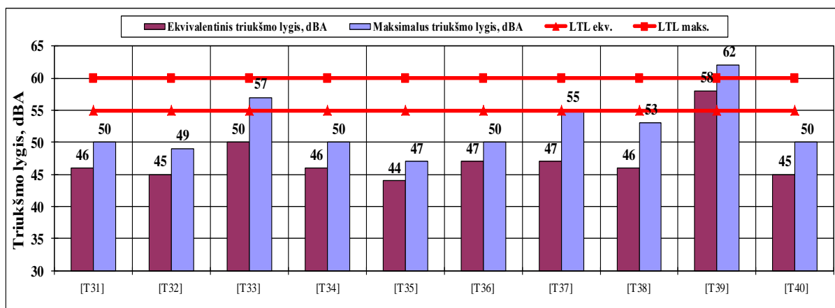
4.26 pav. Ekvivalentiniai ir maksimalūs triukšmo lygiai vakaro metu T31–T40 tyrimo vietose
