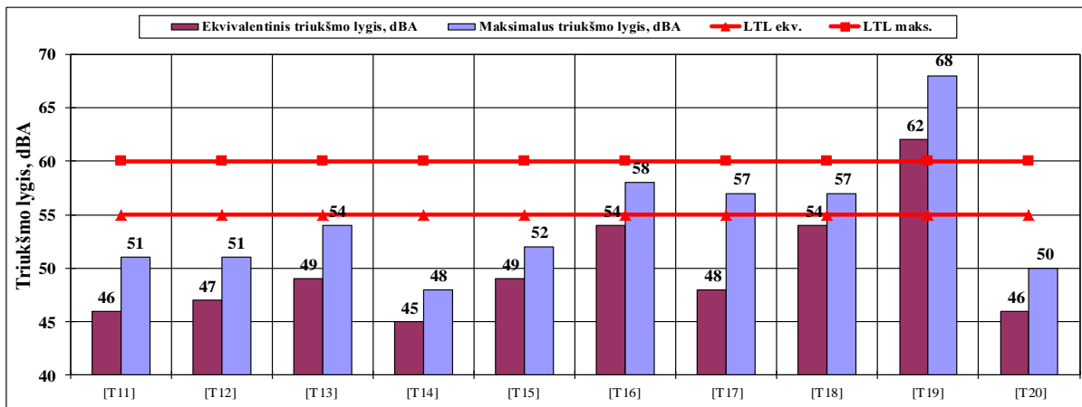
4.24 pav. Ekvivalentiniai ir maksimalūs triukšmo lygiai nakties metu T11–T20 tyrimo vietose
