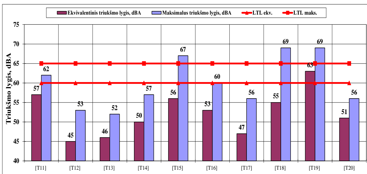
4.8 pav. Ekvivalentiniai ir maksimalūs triukšmo lygiai vakaro metu T11–T20 tyrimo vietose
