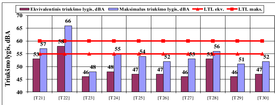
4.25 pav. Ekvivalentiniai ir maksimalūs triukšmo lygiai vakaro metu T21–T30 tyrimo vietose
