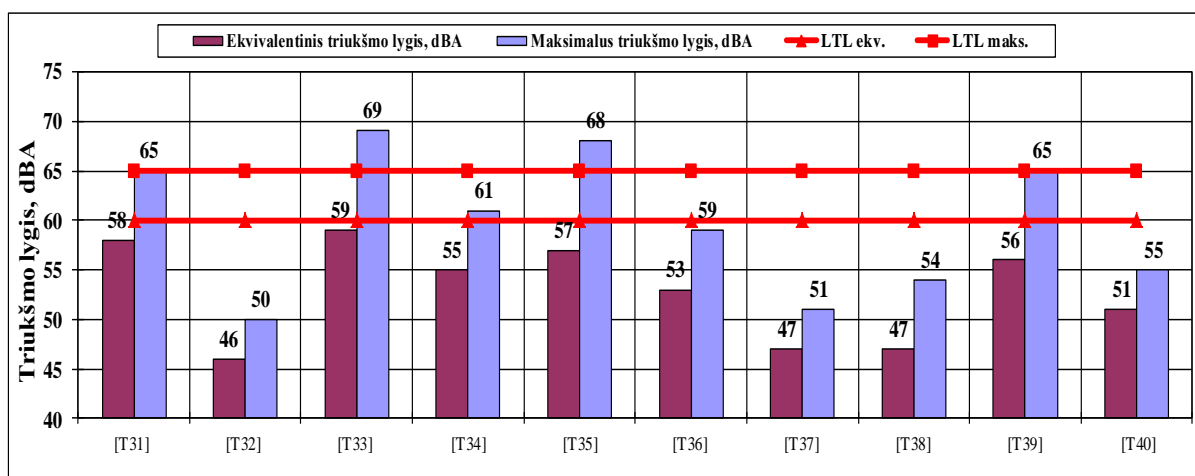
4.22 pav. Ekvivalentiniai ir maksimalūs triukšmo lygiai vakaro metu T31–T40 tyrimo vietose
