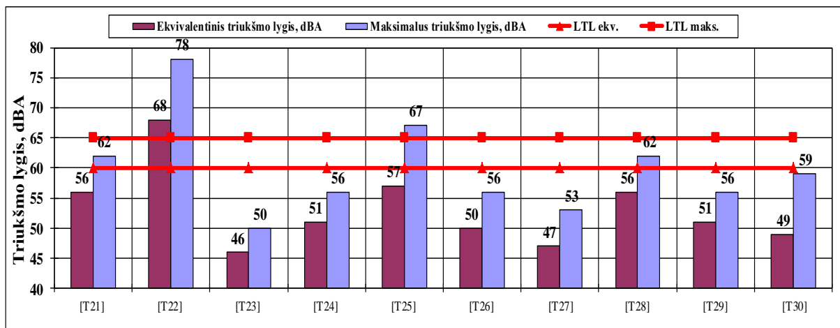
4.21 pav. Ekvivalentiniai ir maksimalūs triukšmo lygiai vakaro metu T21–T30 tyrimo vietose
