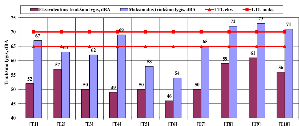
4.3 pav. Ekvivalentiniai ir maksimalūs triukšmo lygiai dienos metu T1–T10 tyrimo vietose
