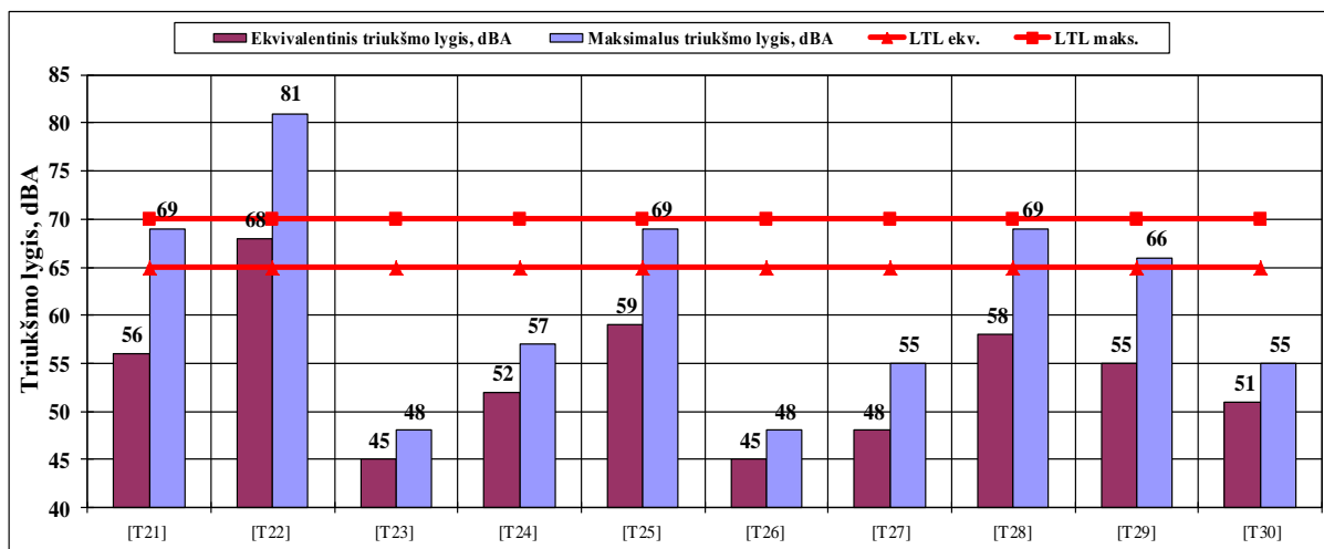
4.17 pav. Ekvivalentiniai ir maksimalūs triukšmo lygiai dienos metu T21–T30 tyrimo vietose
