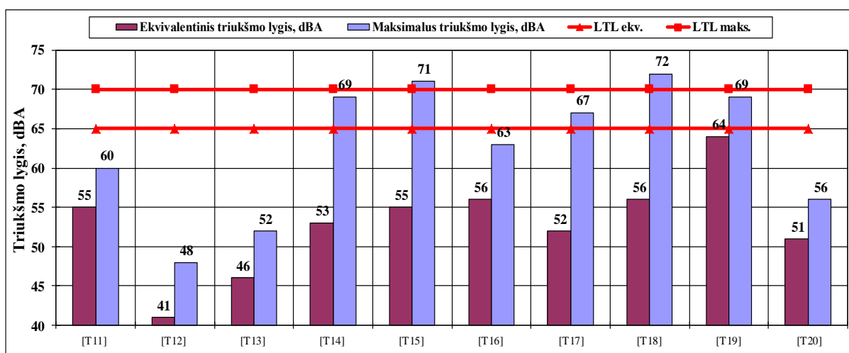
4.16 pav. Ekvivalentiniai ir maksimalūs triukšmo lygiai dienos metu T11–T20 tyrimo vietose
