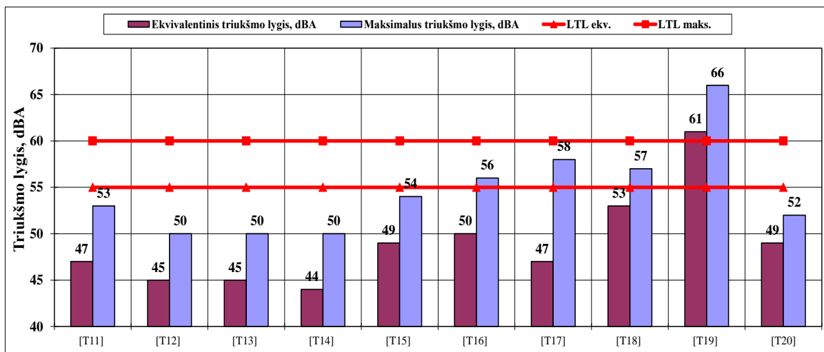
4.12 pav. Ekvivalentiniai ir maksimalūs triukšmo lygiai nakties metu T11–T20 tyrimo vietose
