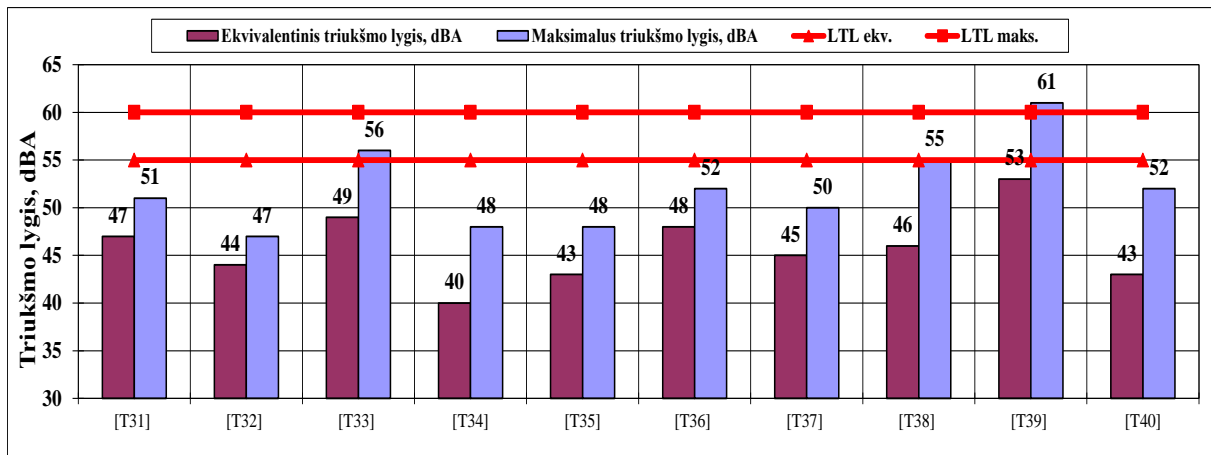
4.14 pav. Ekvivalentiniai ir maksimalūs triukšmo lygiai vakaro metu T31–T40 tyrimo vietose
