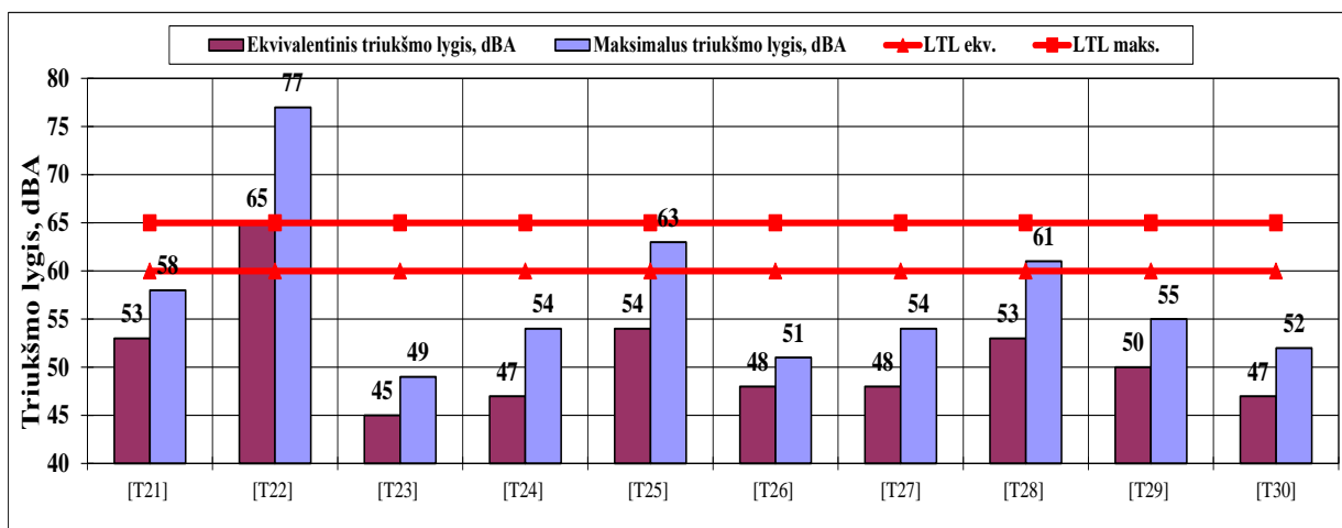
4.9 pav. Ekvivalentiniai ir maksimalūs triukšmo lygiai vakaro metu T21–T30 tyrimo vietose
