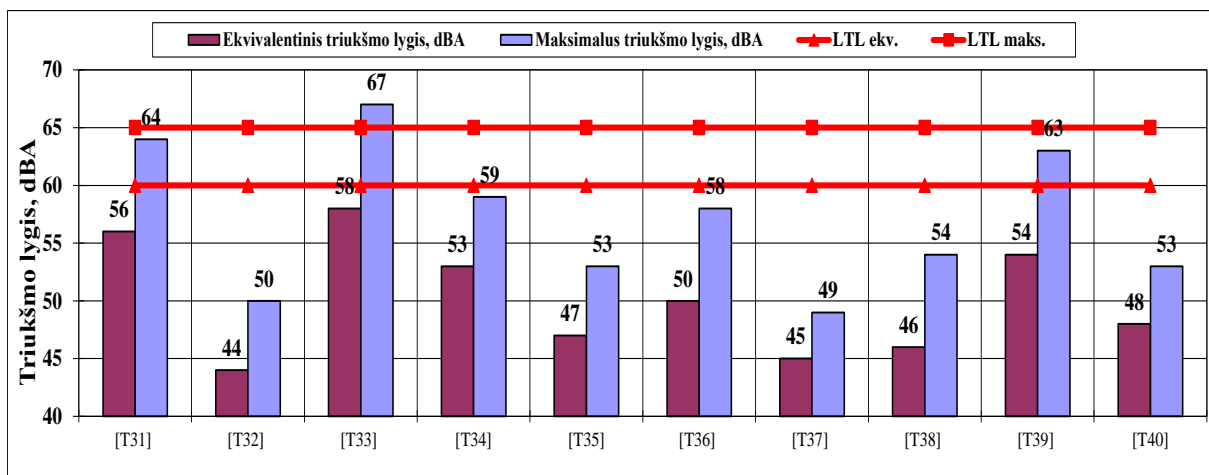
4.10 pav. Ekvivalentiniai ir maksimalūs triukšmo lygiai vakaro metu T31–T40 tyrimo vietose
