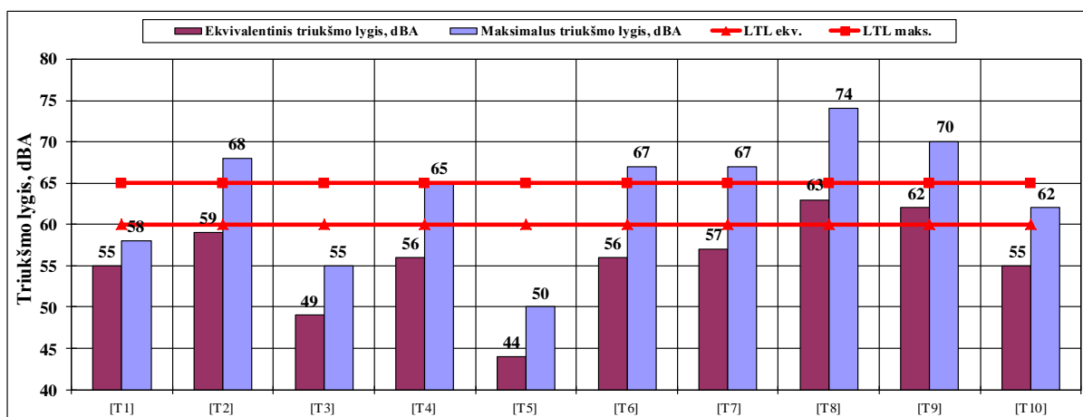
4.19 pav. Ekvivalentiniai ir maksimalūs triukšmo lygiai vakaro metu T1–T10 tyrimo vietose
