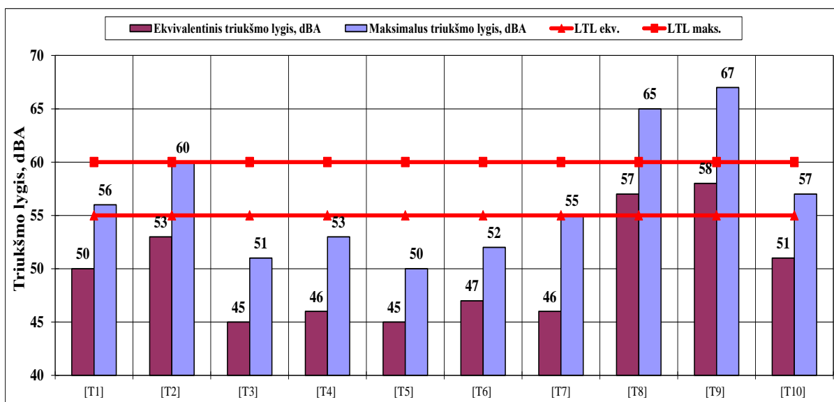
4.11 pav. Ekvivalentiniai ir maksimalūs triukšmo lygiai nakties metu T1–T10 tyrimo vietose
