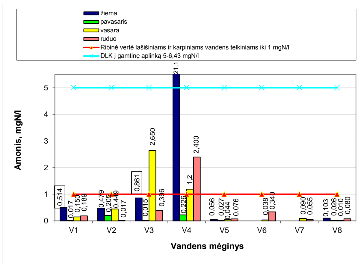
2.11 pav. Amonis paviršiniame vandens telkinyje (pažymėti mėginiai buvo po ledu)
