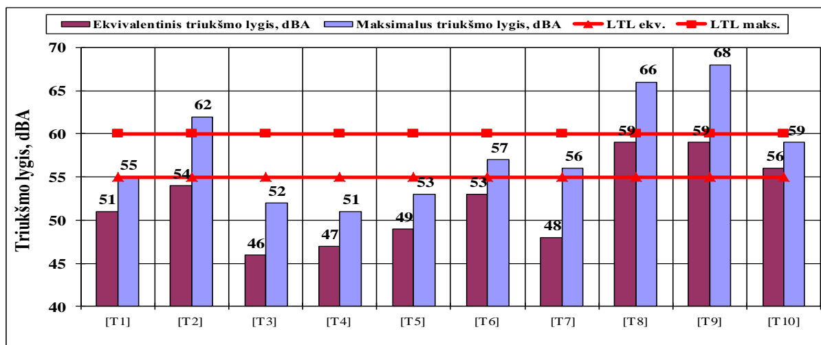
4.23 pav. Ekvivalentiniai ir maksimalūs triukšmo lygiai nakties metu T1–T10 tyrimo vietose
