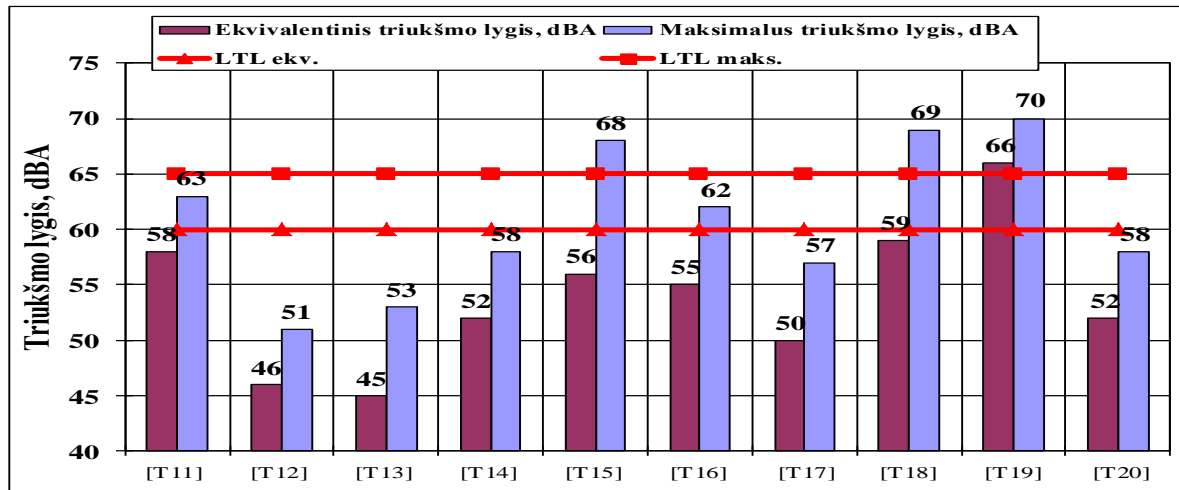
4.20 pav. Ekvivalentiniai ir maksimalūs triukšmo lygiai vakaro metu T11–T20 tyrimo vietose
