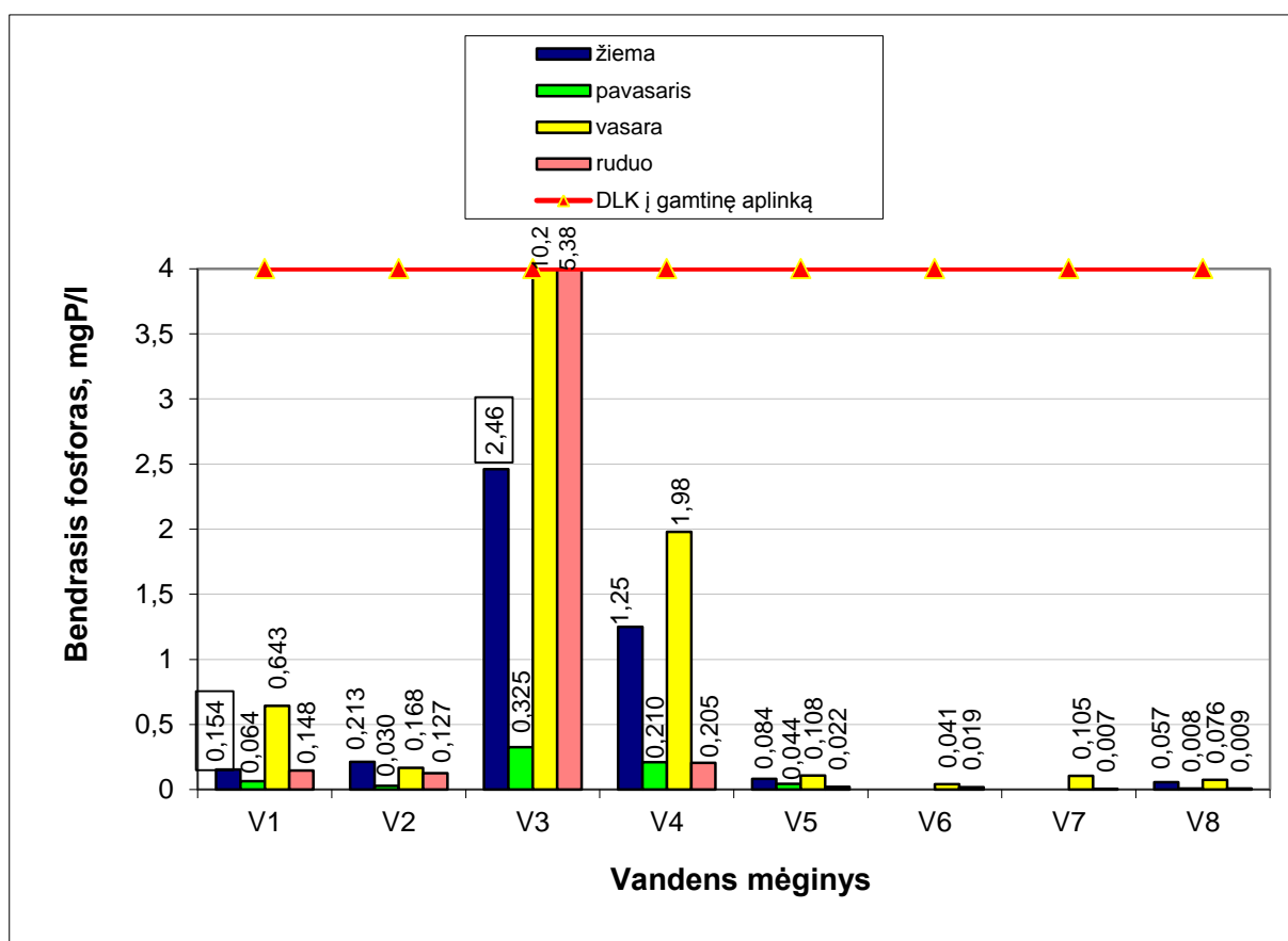
2.12 pav. Bendrasis fosforas paviršiniame vandens telkinyje (pažymėti mėginiai buvo po ledu)
