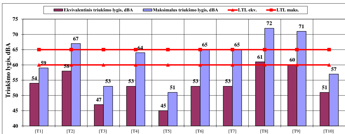
4.7 pav. Ekvivalentiniai ir maksimalūs triukšmo lygiai vakaro metu T1–T10 tyrimo vietose
