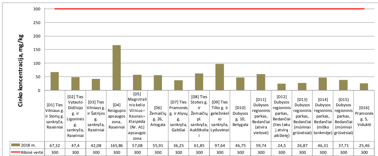
4.8 pav. Cinko (Zn) koncentracija dirvožemyje Raseinių rajone
