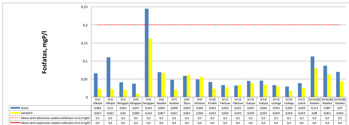
2.8 pav. Fosfatas paviršiniame vandens telkinyje
