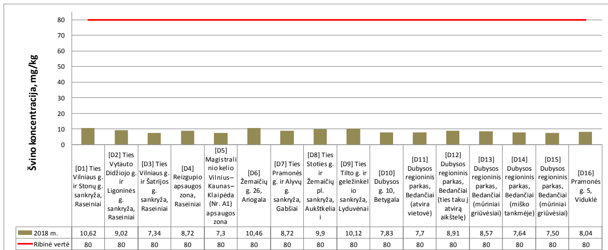
4.7 pav. Švino (Pb) koncentracija dirvožemyje Raseinių rajone
