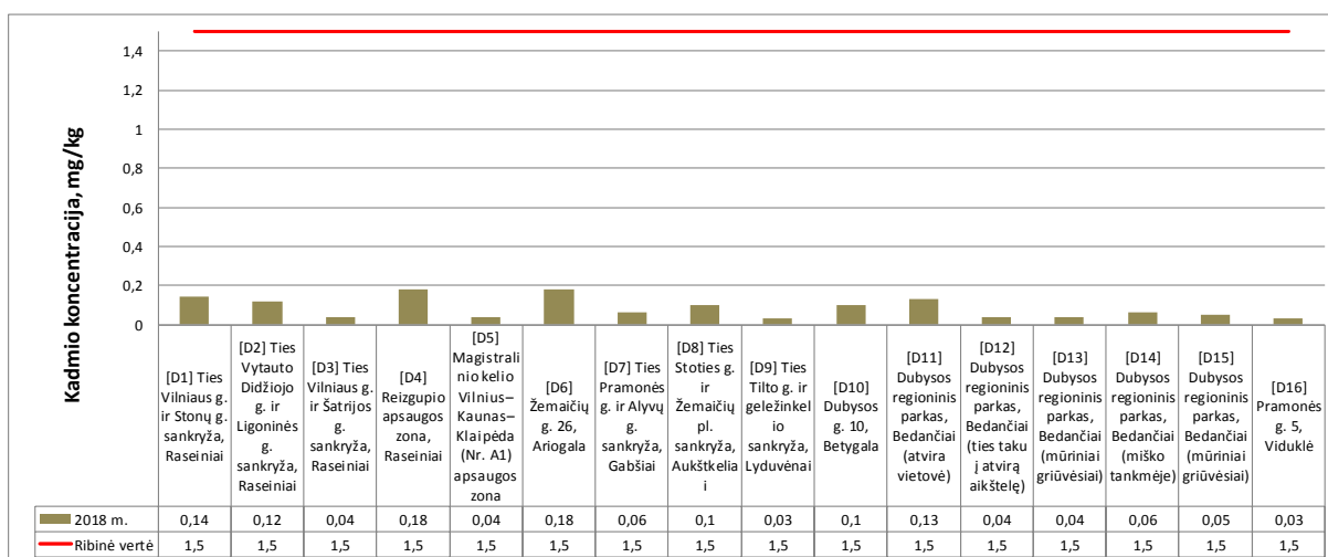
4.3 pav. Kadmio (Cd) koncentracija dirvožemyje Raseinių rajone
