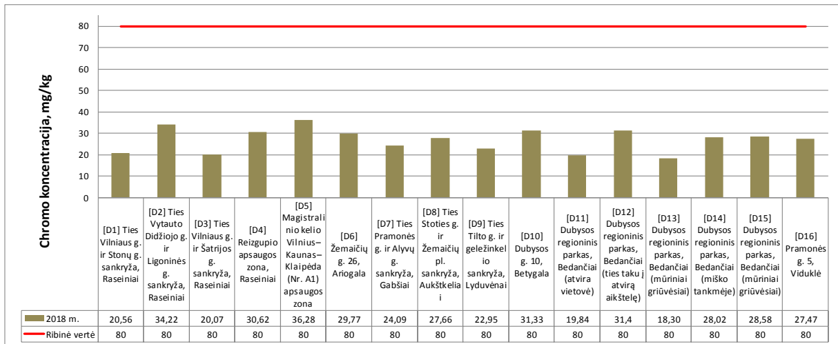
4.4 pav. Chromo (Cr) koncentracija dirvožemyje Raseinių rajone
