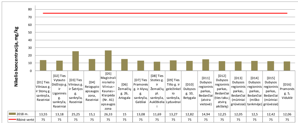
4.6 pav. Nikelio (Ni) koncentracija dirvožemyje Raseinių rajone
