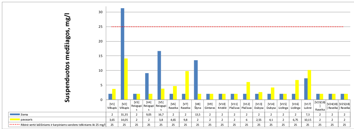
2.6 pav. Suspensijos medžiagos paviršiniame vandens telkinyje
