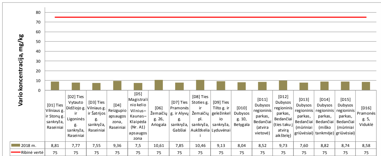
4.5 pav. Vario (Cu) koncentracija dirvožemyje Raseinių rajone
