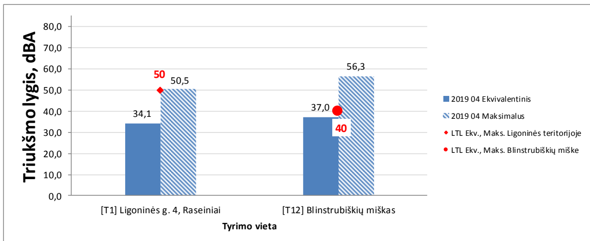
3.8 pav. Ekvivalentiniai ir maksimalūs triukšmo lygiai nakties metu, tyliosiose zonos
