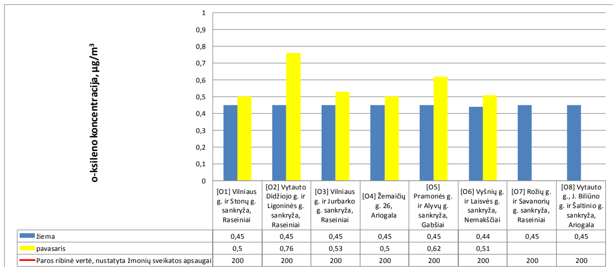
1.10 pav. o-ksilenų paros koncentracija aplinkos ore Raseinių rajone (o-ksilenų paros ribinė vertė, nustatyta žmonių sveikatos apsaugai (200 µg/m³))
