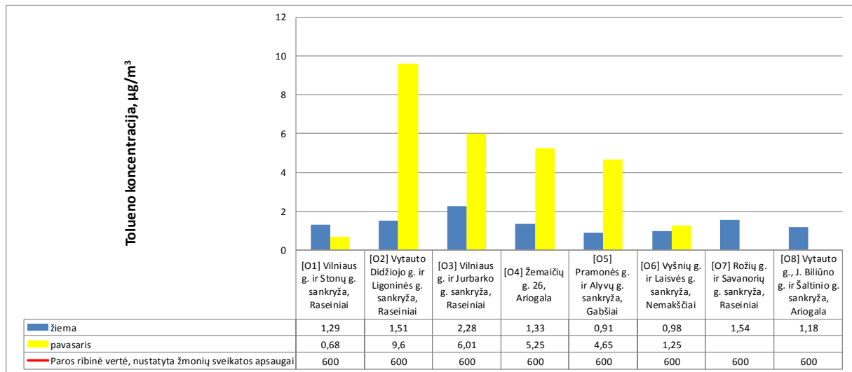
1.7 pav. Tolueno paros koncentracija aplinkos ore Raseinių rajone (tolueno paros ribinė vertė, nustatyta žmonių sveikatos apsaugai ( 600 \mu\text{g}/\text{m}^3 ))
