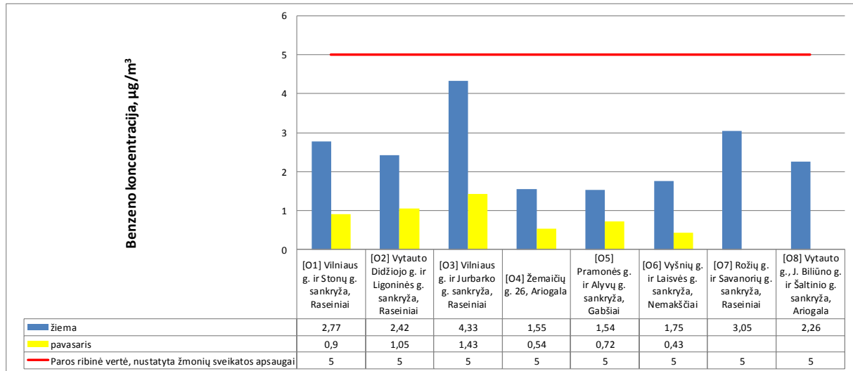
1.6 pav. Benzeno paros koncentracija aplinkos ore Raseinių rajone (benzeno paros ribinė vertė, nustatyta žmonių sveikatos apsaugai ( 5 \mu\text{g}/\text{m}^3 ))
