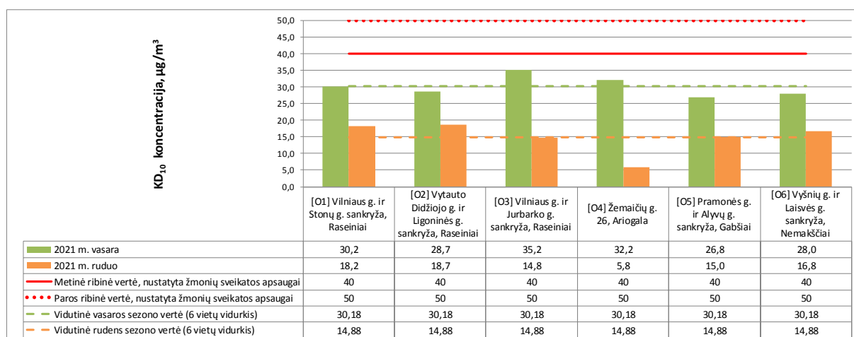
1.5 pav. Kietųjų dalelių ( \text{KD}_{10} ) koncentracija aplinkos ore Raseinių rajone (paros ribinė vertė, nustatyta žmonių sveikatos apsaugai – 50 \mu\text{g}/\text{m}^3 ir metinė ribinė vertė, nustatyta žmonių sveikatos apsaugai – 40 \mu\text{g}/\text{m}^3 )
