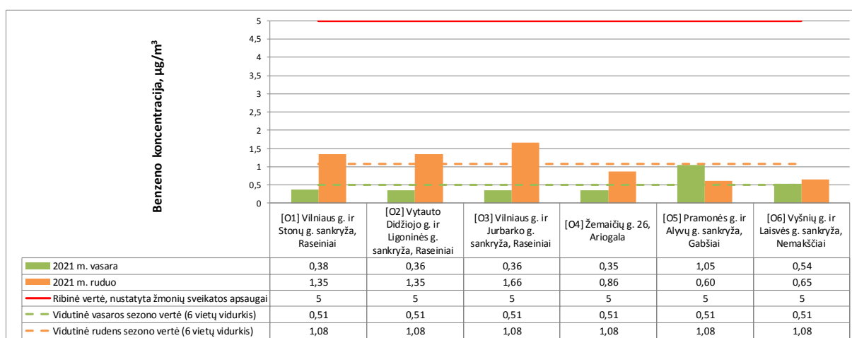
1.6 pav. Benzono koncentracija aplinkos ore Raseinių rajone (benzeno paros ribinė vertė, nustatyta žmonių sveikatos apsaugai – 5 \mu\text{g}/\text{m}^3 )
