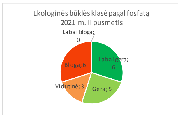
2.11 pav. Ekologinės būklės klasė pagal fosfatą. 2021 m. II pusmečio apibendrinimas
