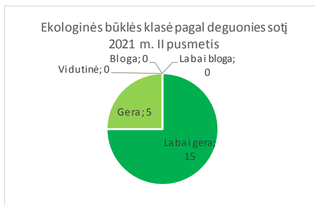
2.6 pav. Ekologinės būklės klasė pagal deguonies sotį. 2021 m. II pusmečio apibendrinimas
