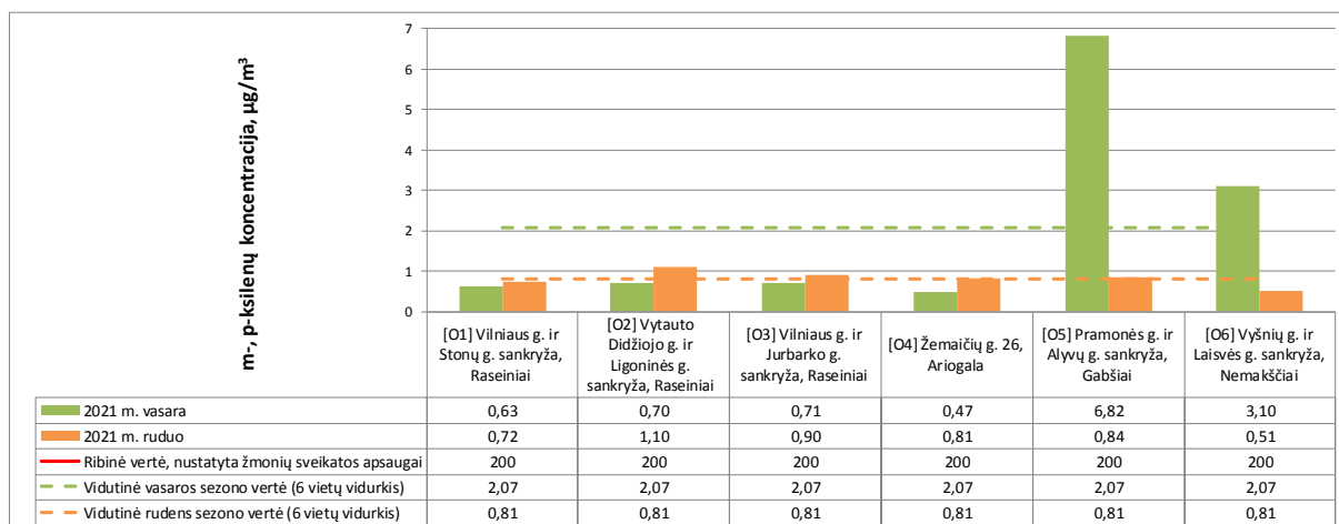
1.9 pav. m-, p-ksilenų koncentracija aplinkos ore Raseinių rajone (m-, p-ksilenų paros ribinė vertė, nustatyta žmonių sveikatos apsaugai – 200 µg/m 3 )
