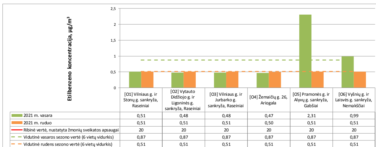
1.8 pav. Etilbenzeno koncentracija aplinkos ore Raseinių rajone (etilbenzeno paros ribinė vertė, nustatyta žmonių sveikatos apsaugai – 20 µg/m 3 )
