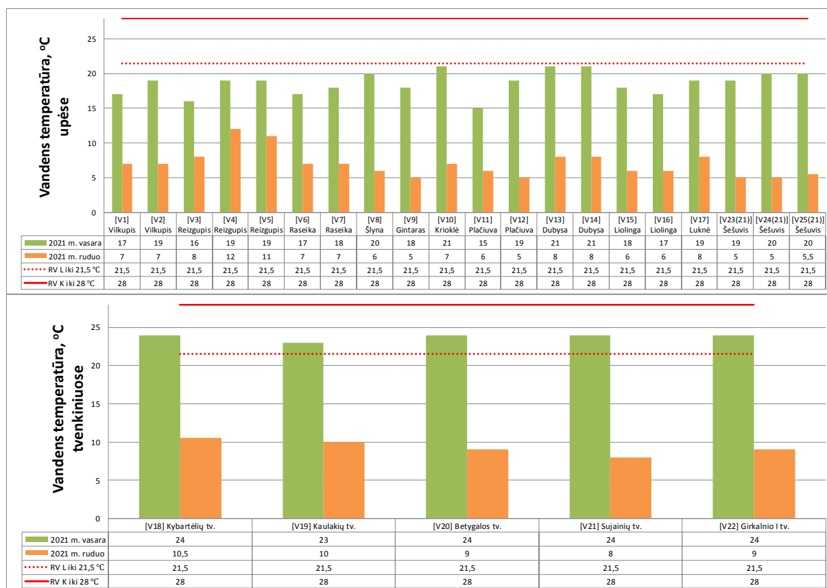
2.4 pav. Paviršinio vandens telkinio temperatūra (RV L – ribinė vertė lašišiniams vandens telkiniams iki 21,5 °C, RV K – ribinė vertė karpiniams vandens telkiniams iki 28 °C)
