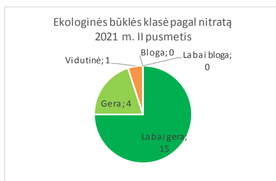
2.14 pav. Ekologinės būklės klasė pagal nitratą. 2021 m. II pusmečio apibendrinimas
