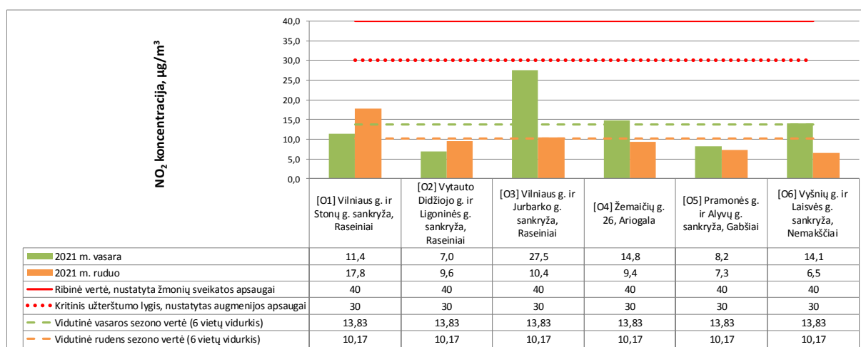
1.4 pav. Azoto dioksido ( \text{NO}_2 ) koncentracija aplinkos ore Raseinių rajone (metinė ribinė vertė, nustatyta žmonių sveikatos apsaugai – 40 \mu\text{g}/\text{m}^3 ir metinis kritinis taršos lygis, nustatytas augmenijos apsaugai – 30 \mu\text{g}/\text{m}^3 )
