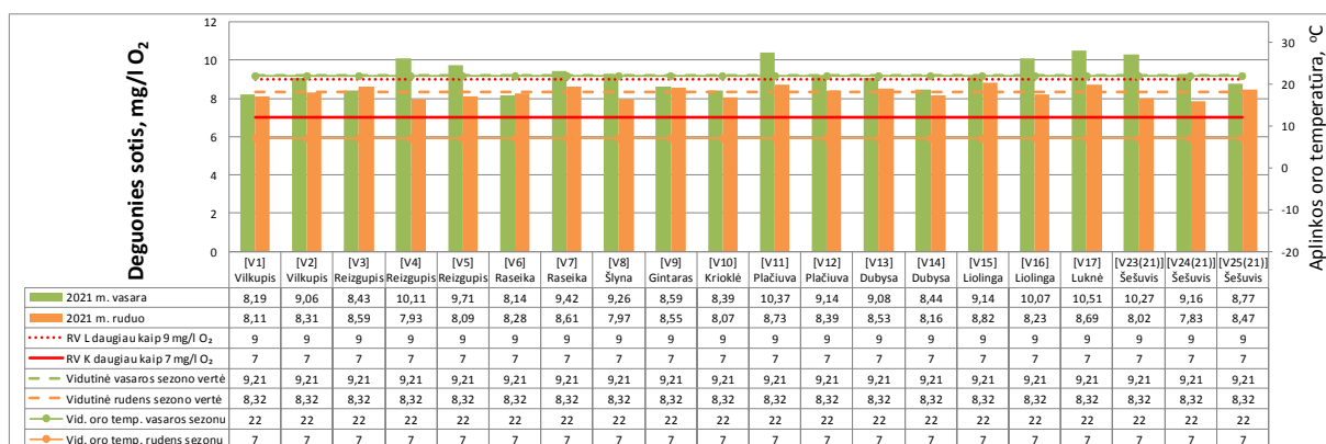
2.5 pav. Deguonies sotis paviršiniame vandens telkinyje (RV L – ribinė vertė lašišiniams vandens telkiniams daugiau kaip 9 mg/l O 2 , RV K – ribinė vertė karpiniams vandens telkiniams daugiau kaip 7 mg/l O 2 )
