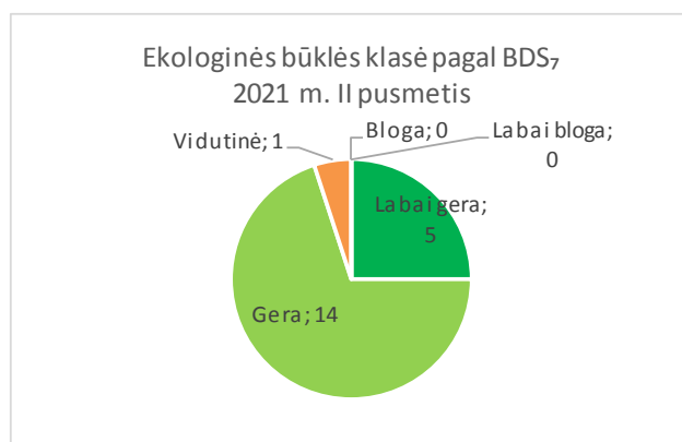
2.9 pav. Ekologinės būklės klasė pagal BDS 7 . 2021 m. II pusmečio apibendrinimas
