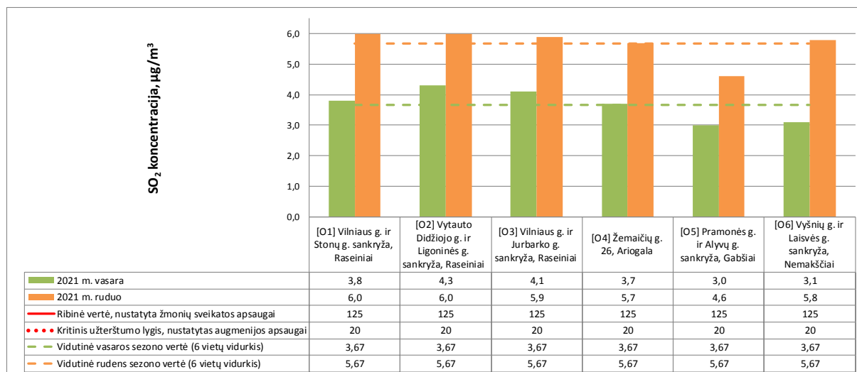
1.3 pav. Sieros dioksido ( \text{SO}_2 ) koncentracija aplinkos ore Raseinių rajone (paros ribinė vertė, nustatyta žmonių sveikatos apsaugai – 125 \mu\text{g}/\text{m}^3 ir metinis kritinis taršos lygis, nustatytas augmenijos apsaugai – 20 \mu\text{g}/\text{m}^3 )
