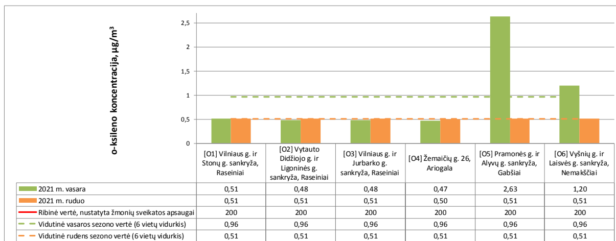
1.10 pav. o-ksileno koncentracija aplinkos ore Raseinių rajone (o-ksileno paros ribinė vertė, nustatyta žmonių sveikatos apsaugai – 200 µg/m³)
