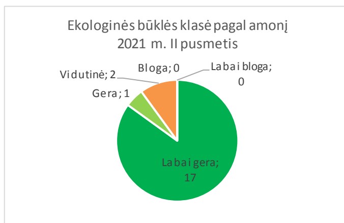
2.16 pav. Ekologinės būklės klasė pagal amonį. 2021 m. II pusmečio apibendrinimas
