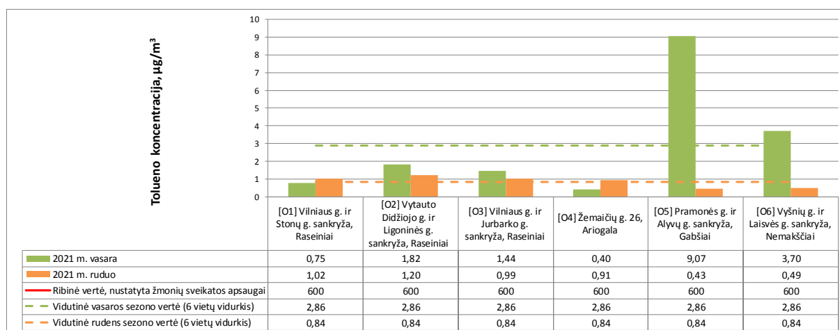
1.7 pav. Tolueno koncentracija aplinkos ore Raseinių rajone (tolueno paros ribinė vertė, nustatyta žmonių sveikatos apsaugai – 600 µg/m³)
